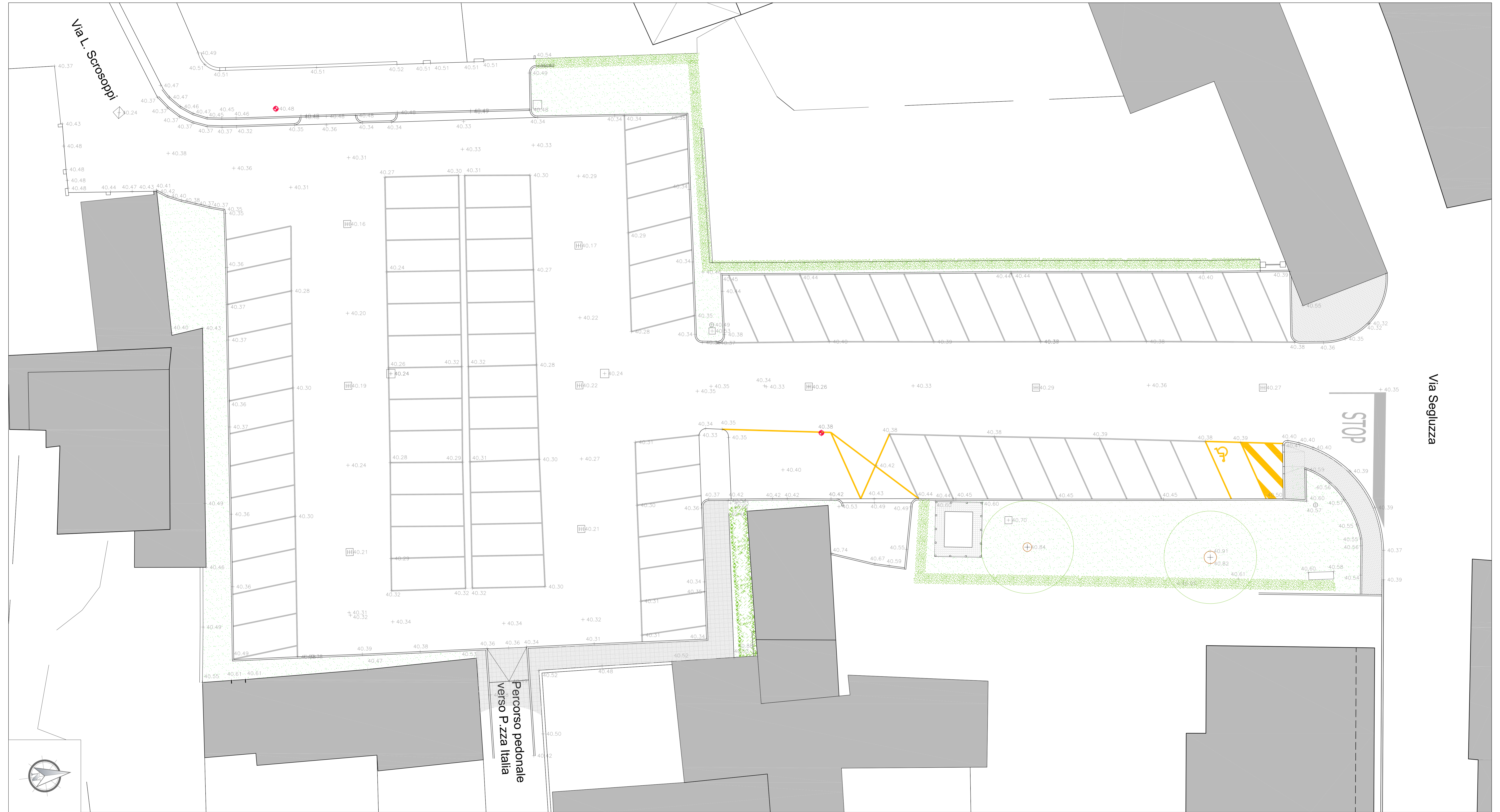
STATO DI PROGETTO: Parcheggio di via Segluzza, Scala 1:100
