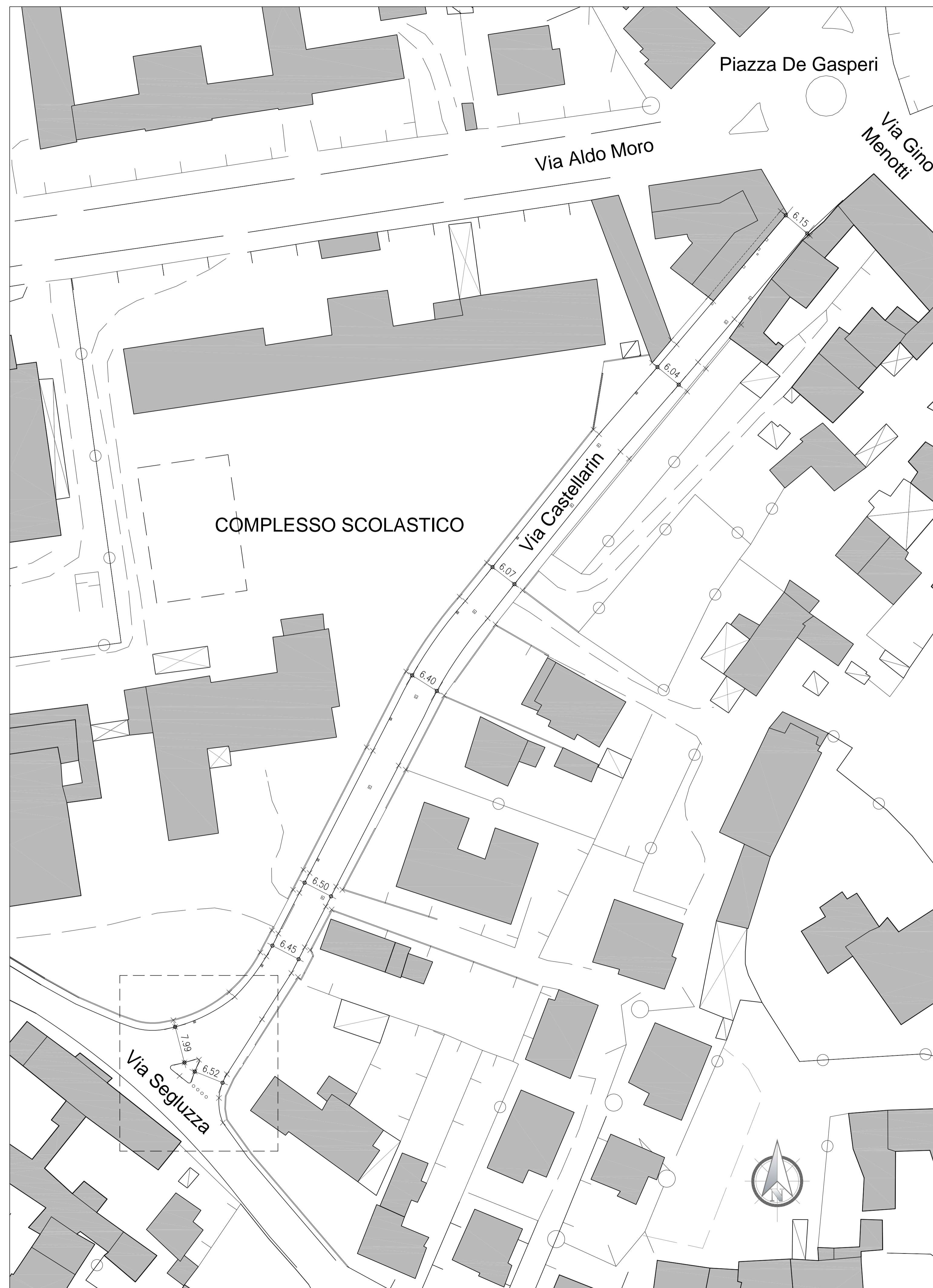
2 - Via Castellarin: Planimetria generale, Scala 1:500
