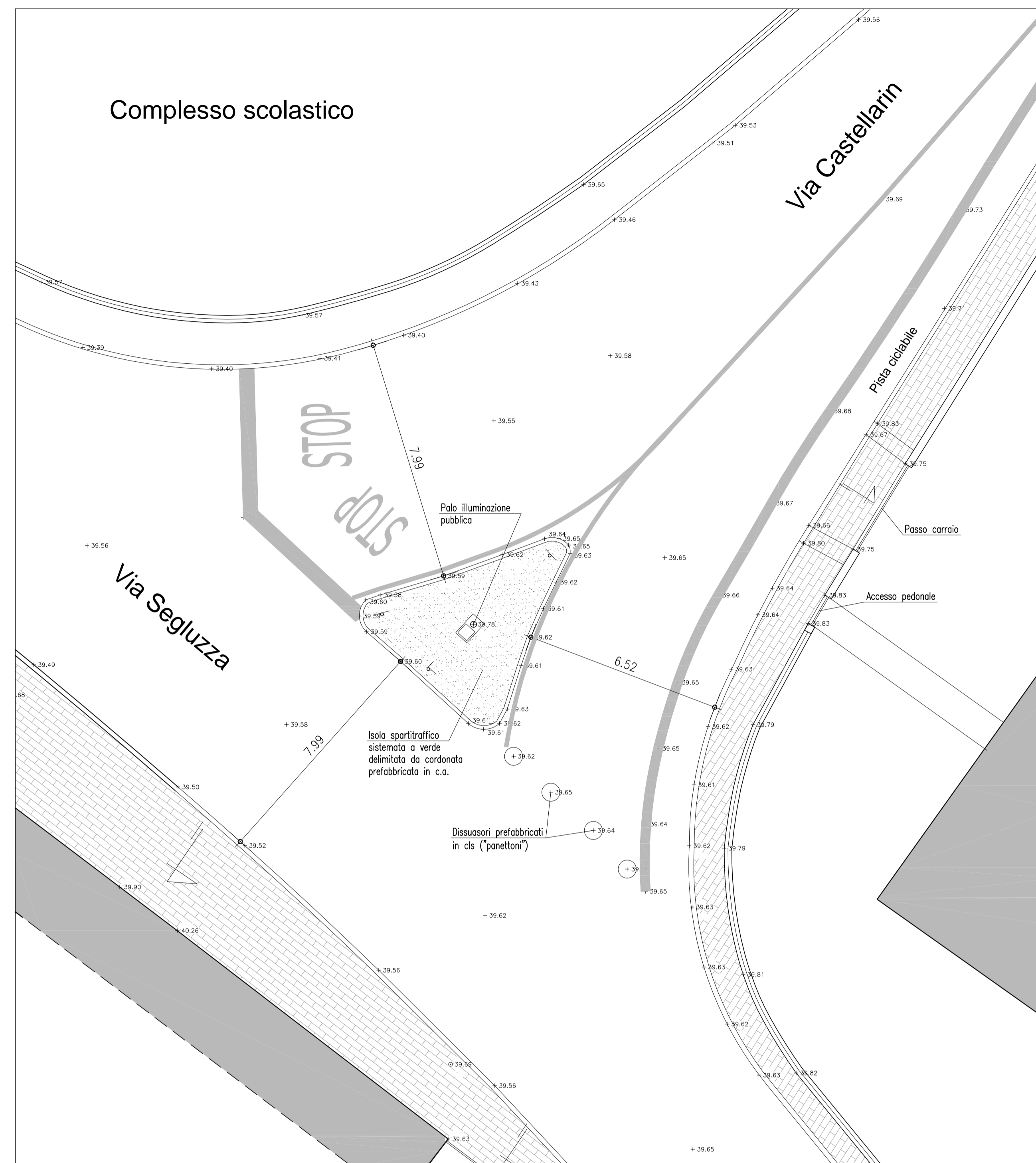
Dettaglio isola spartitraffico incrocio con via Segluza, Scala 1:100
