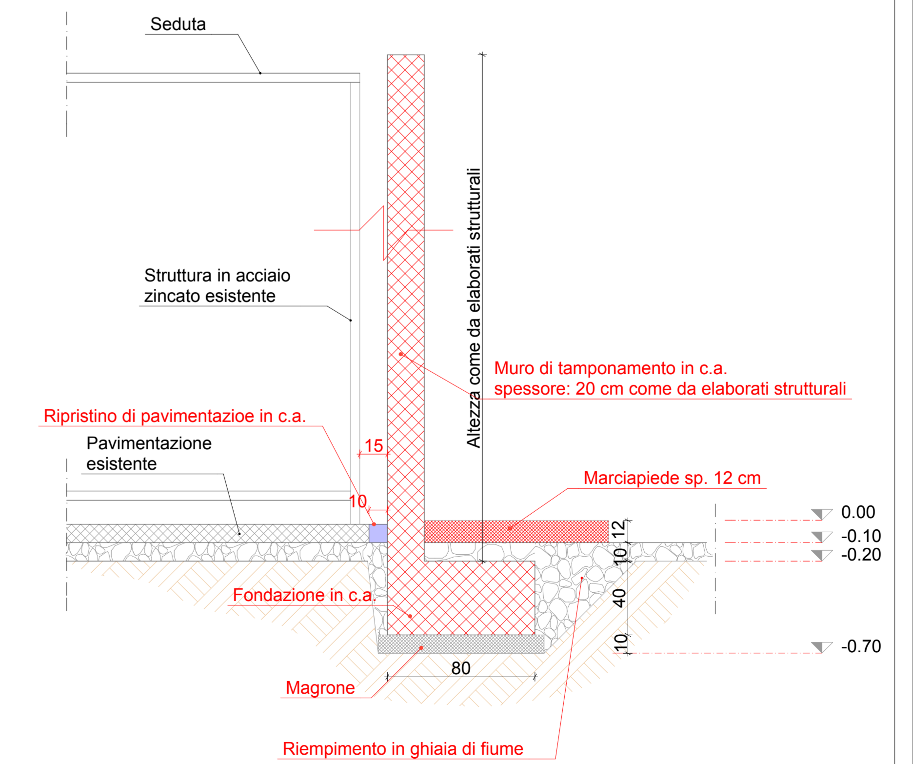
PARTICOLARE PARETE DI TAMPONAMENTO scala 1:20
