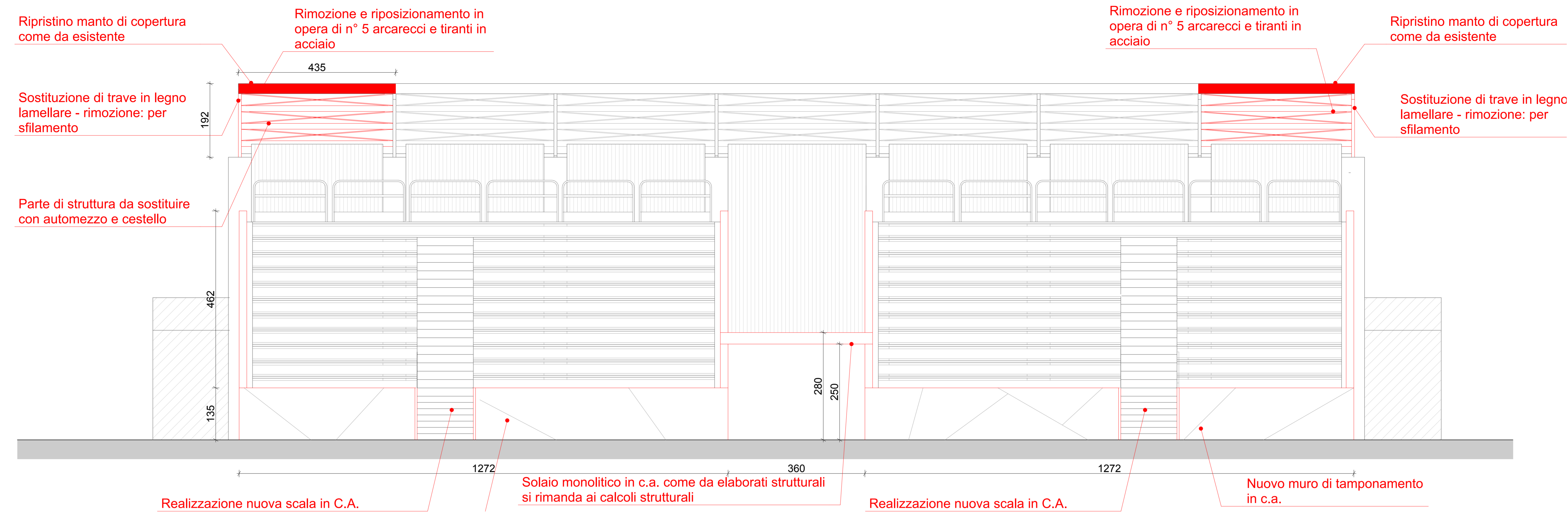
PROSPETTO EST scala 1:50
