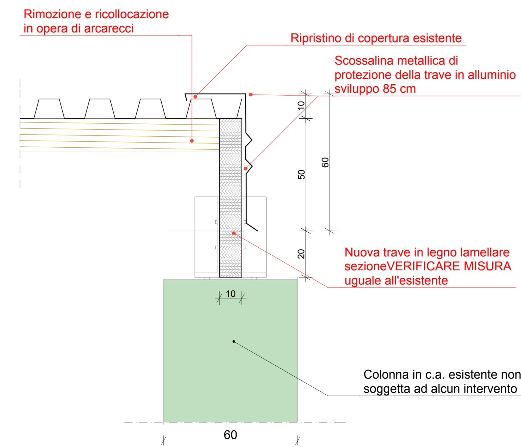
SEZIONE TRAVE scala 1:10
