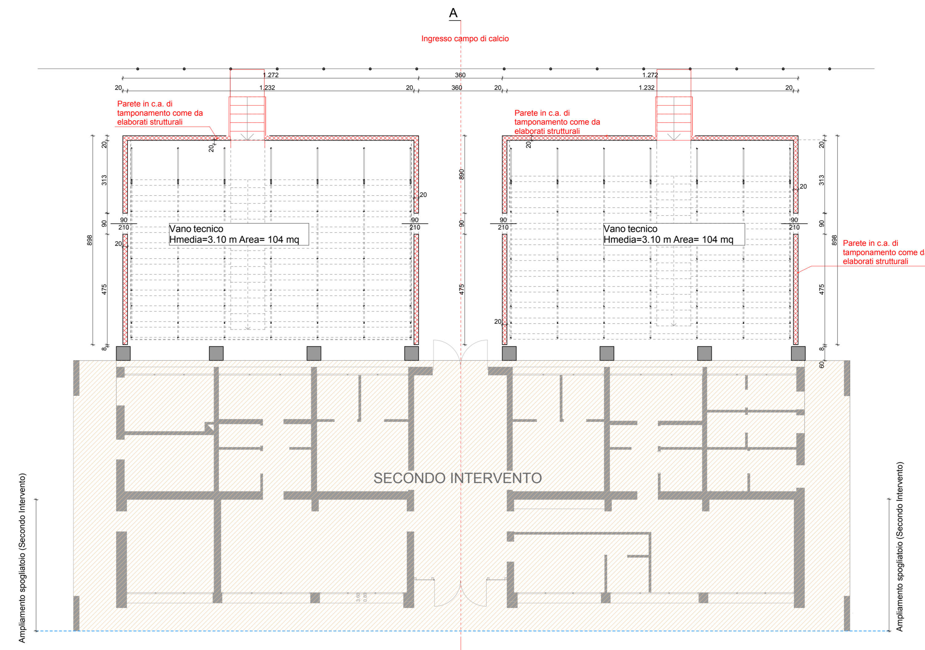
PIANTA SOTTO-TRIBUNE scala 1:100
