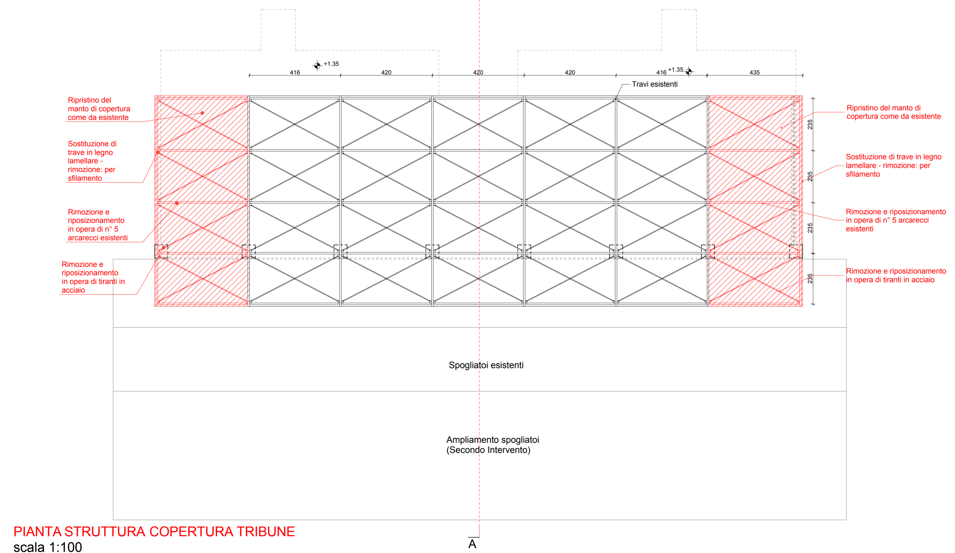
PIANTA TRIBUNE scala 1:100
