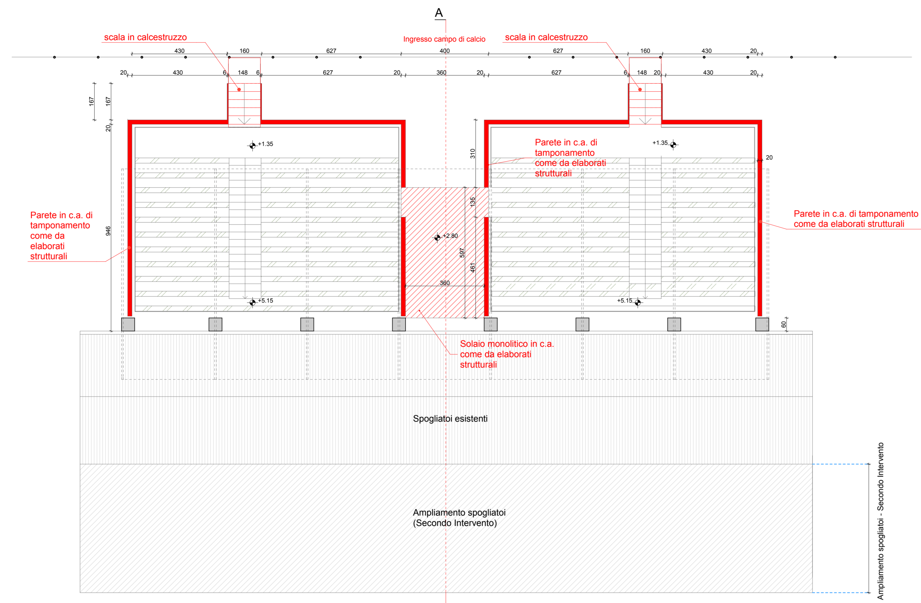
PIANTA TRIBUNE scala 1:100
