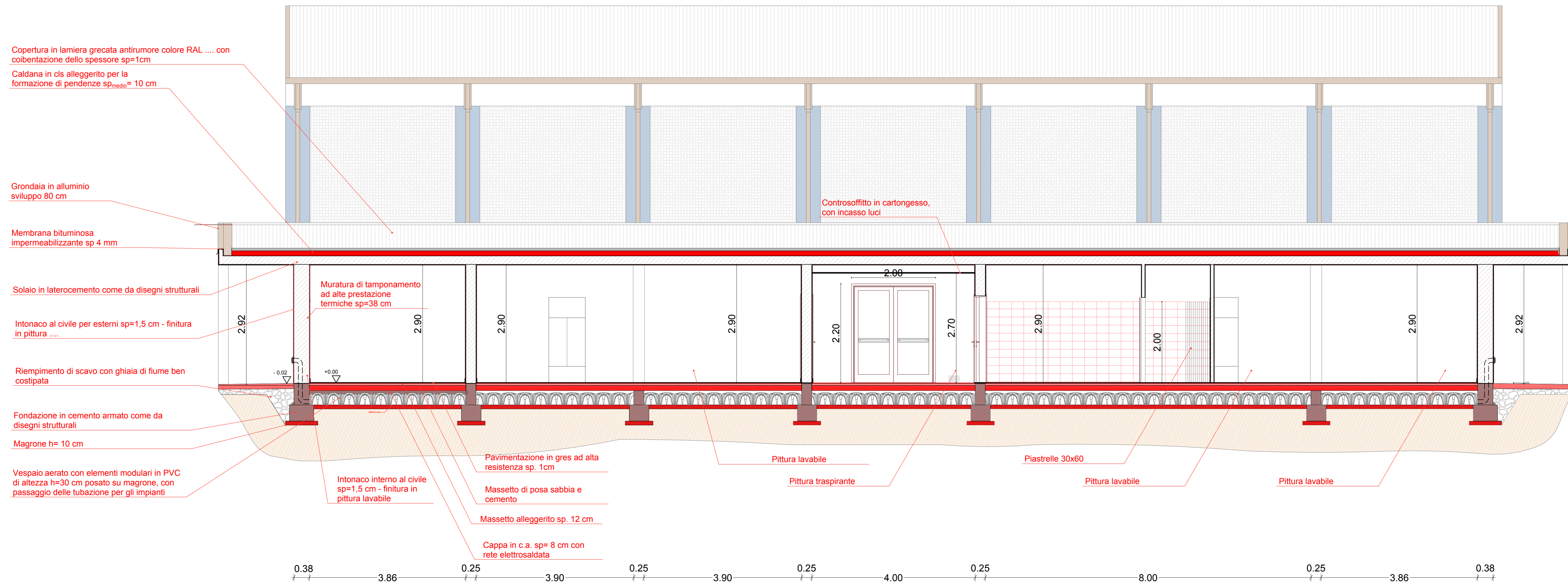
Sezione BB Scala 1:100
