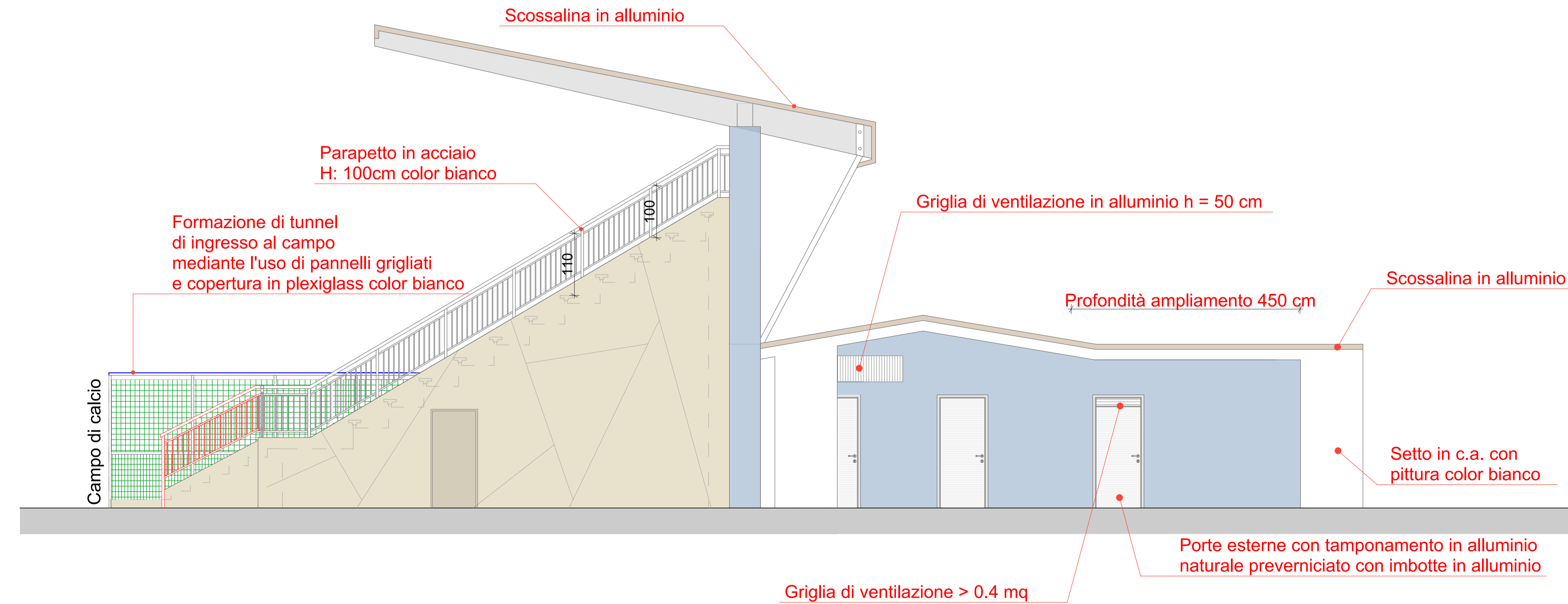
SEZIONE NORD Scala 1:100
