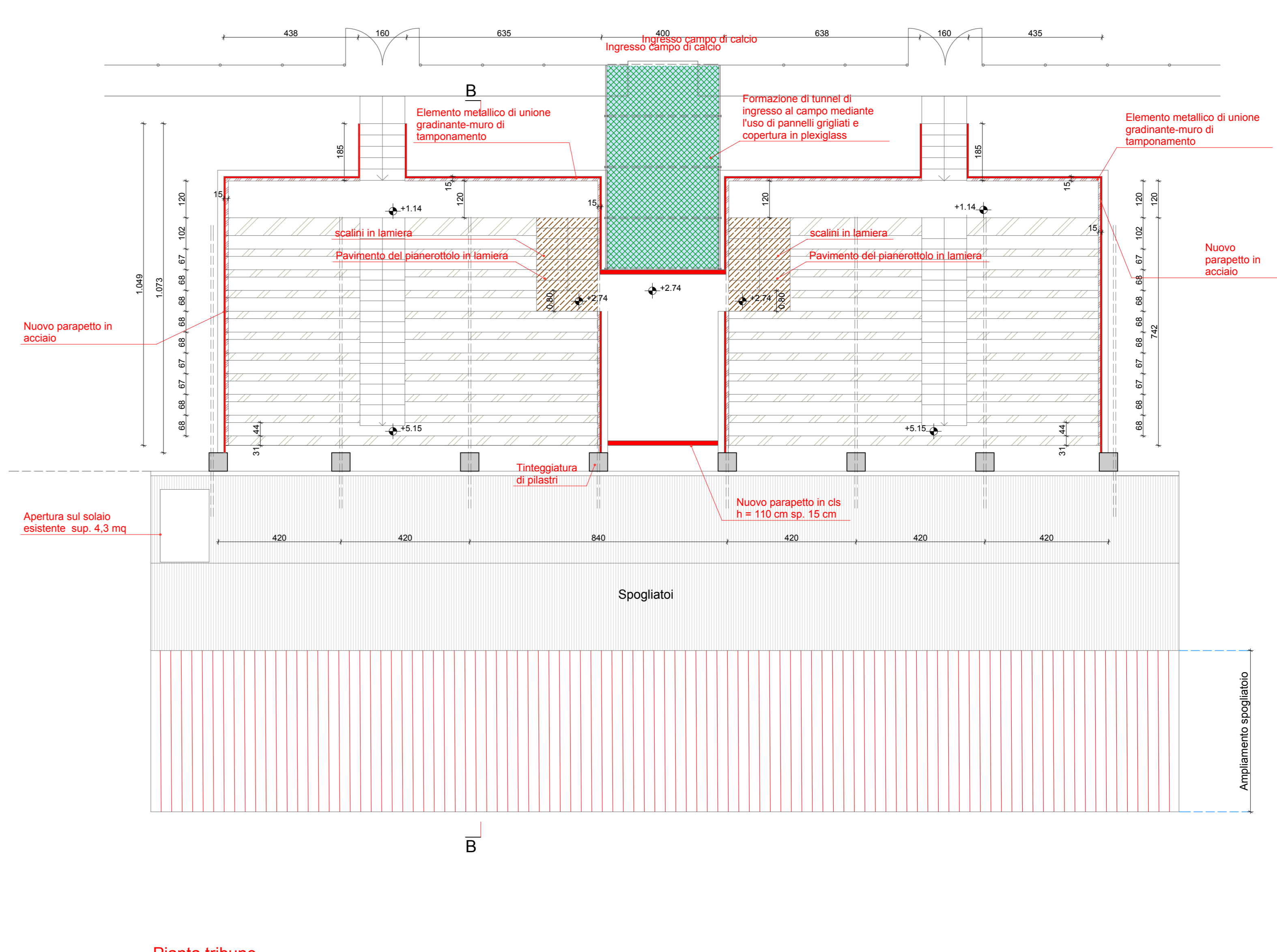
Pianta tribune Scala 1:100
