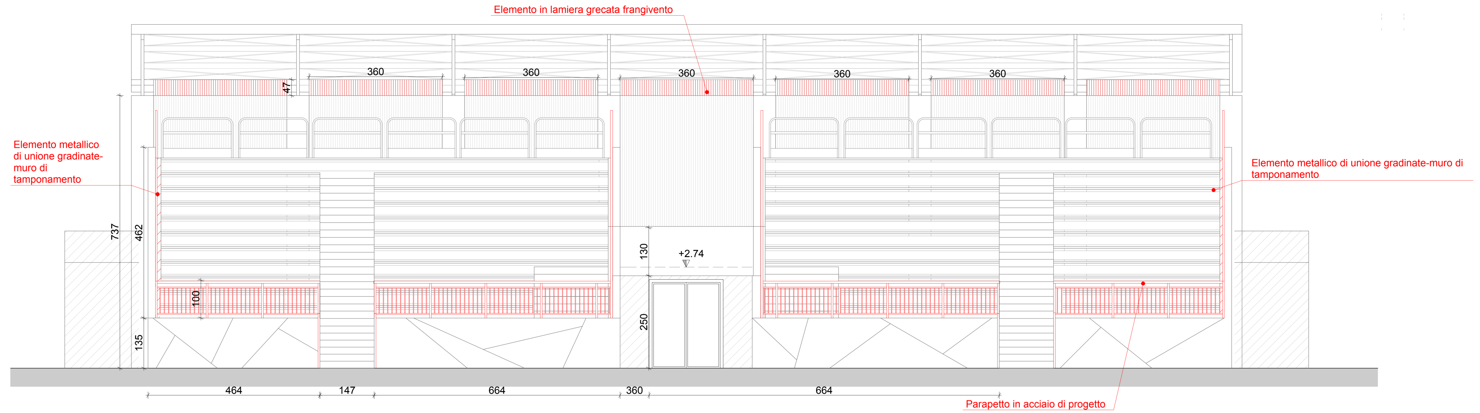
Prospetto NORD Scala 1:50
