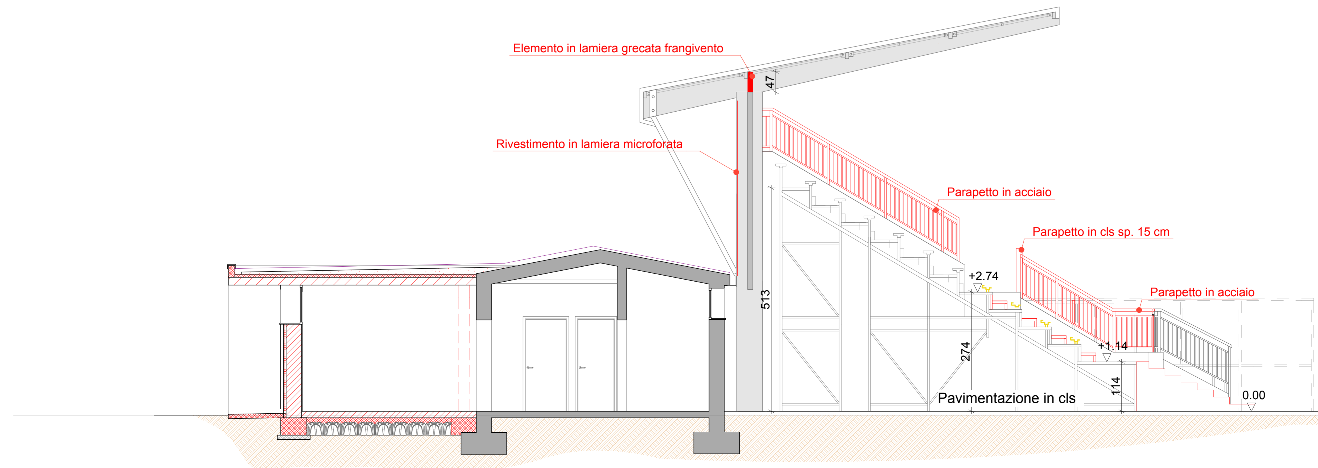
Prospetto SUD Scala 1:50
