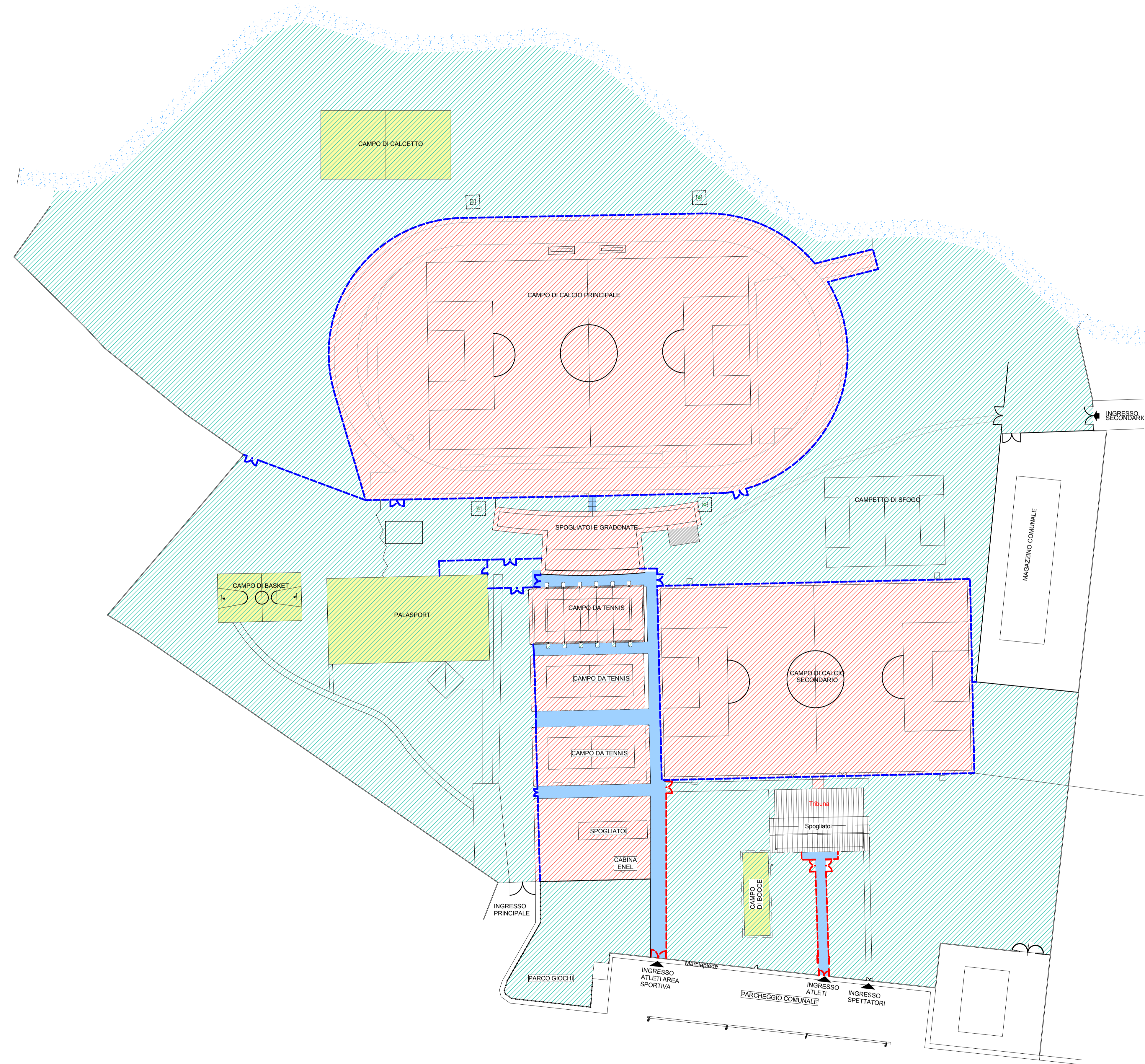
Planimetria scala 1:750
