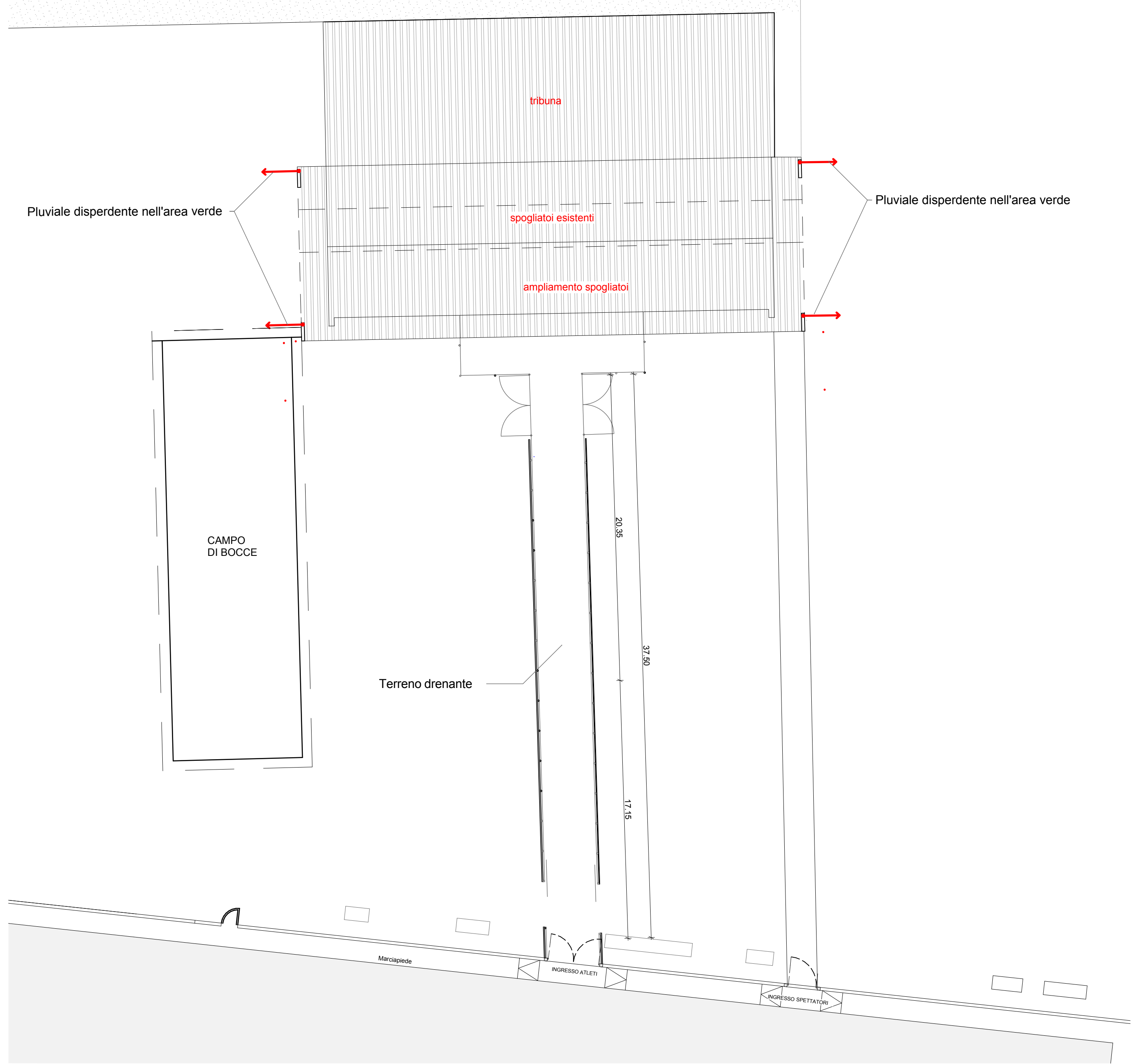
PIANTA RETE FOGNARIA ESTERNA ACQUE METEORICHE SCALA 1:200
