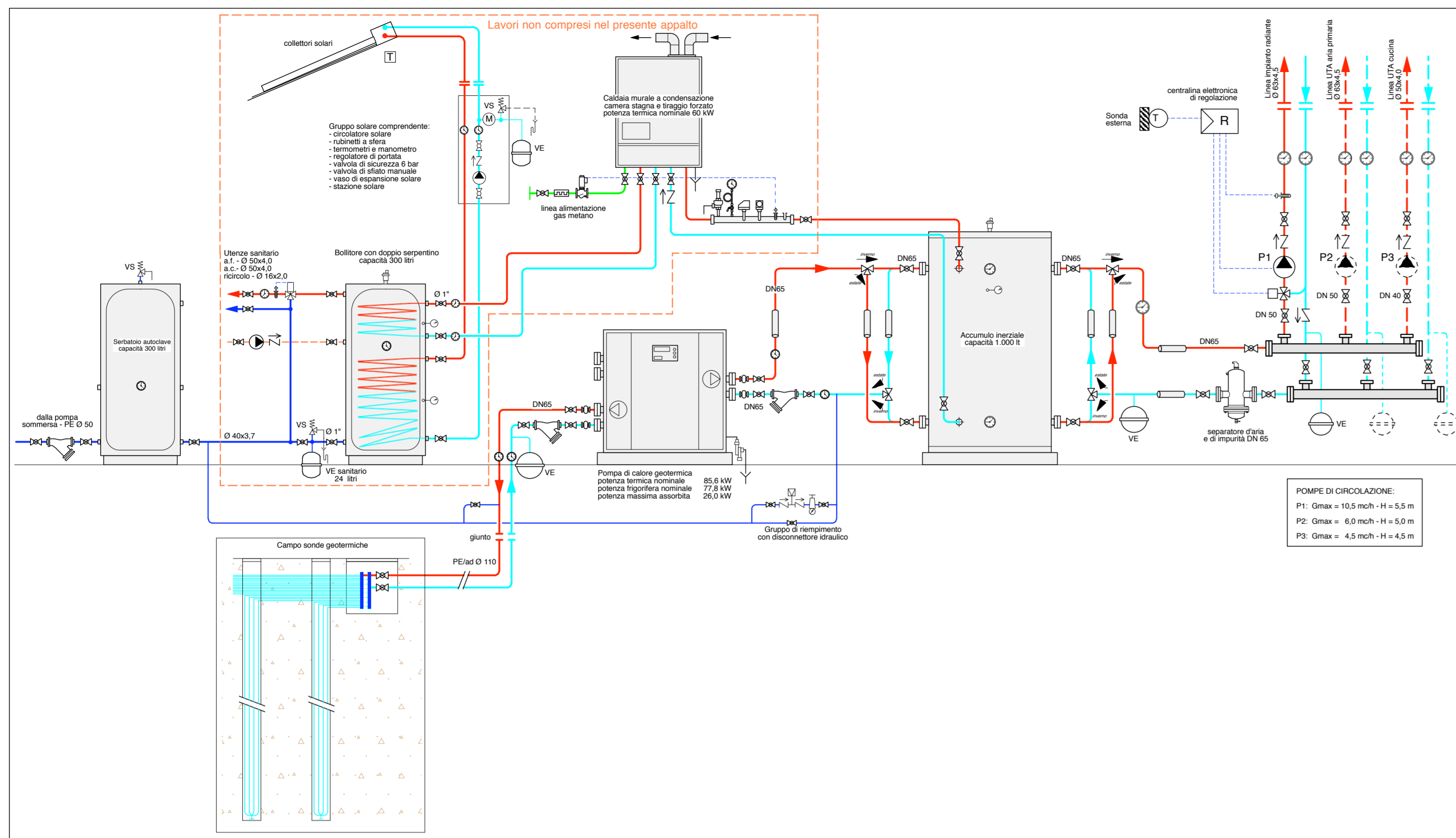
SCHEMA CENTRALE TERMO-FRIGORIFERA
