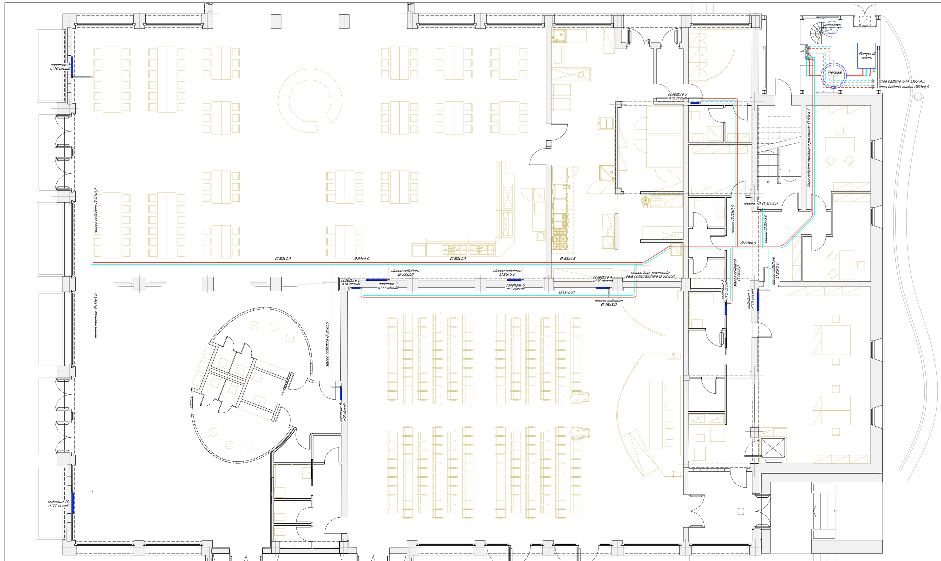
LINEE PRINCIPALI DI DISTRIBUZIONE PIANO TERRA - scala 1:100
